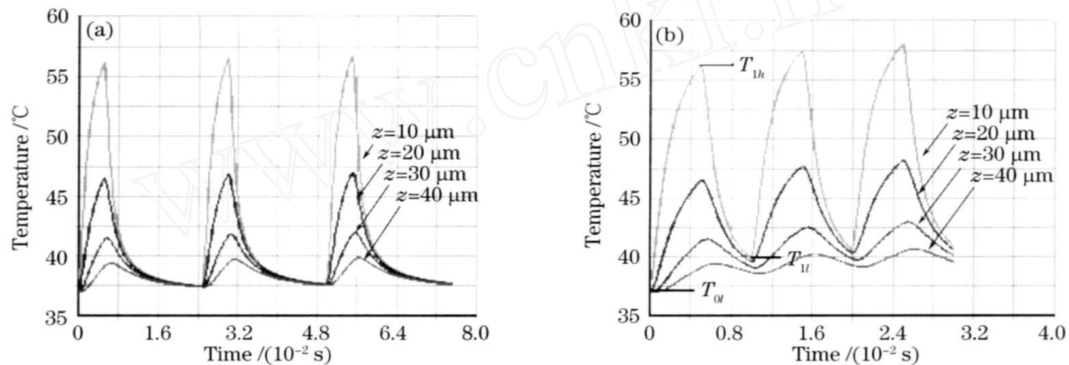
图 4 脉冲间隔为 20\ \text{ms} (a) 和 5\ \text{ms} (b) 组织升温图
