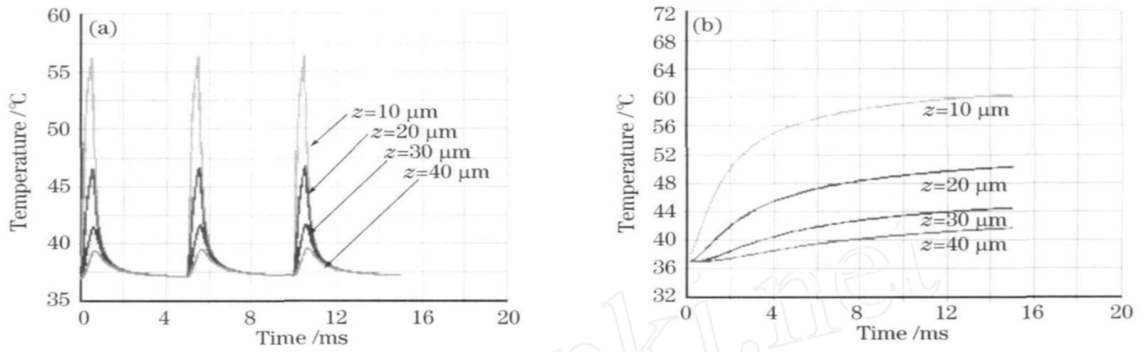
图 1 脉冲激光 (a) 和连续激光 (b) 辐照下皮肤不同深度处的温度随时间的变化
