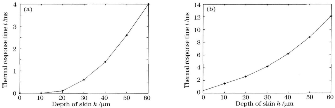
图 2 (a) 组织不同深度处的热响应时间, (b) 组织不同深度处热弛豫时间
