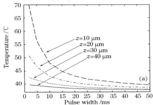
图 3 (a) 不同深度组织升温所达最高温度与脉宽的关系, (b) 评价函数 随脉冲间隔的变化关系
